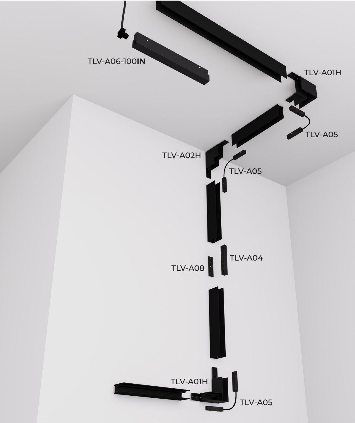
szyna typ H/ track type H szyna natynkowa wysoka (zaślepka w kpl.) high-profile surface track (ends caps incl.)
