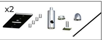
TLV-A07 Pendant Kit do zawieszenia szyn wysokich typu H oraz niskich typu L Suspension KIT for high tracks (type H) and low tracks (type L)
